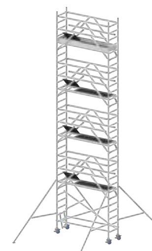
RSS075x245x800
